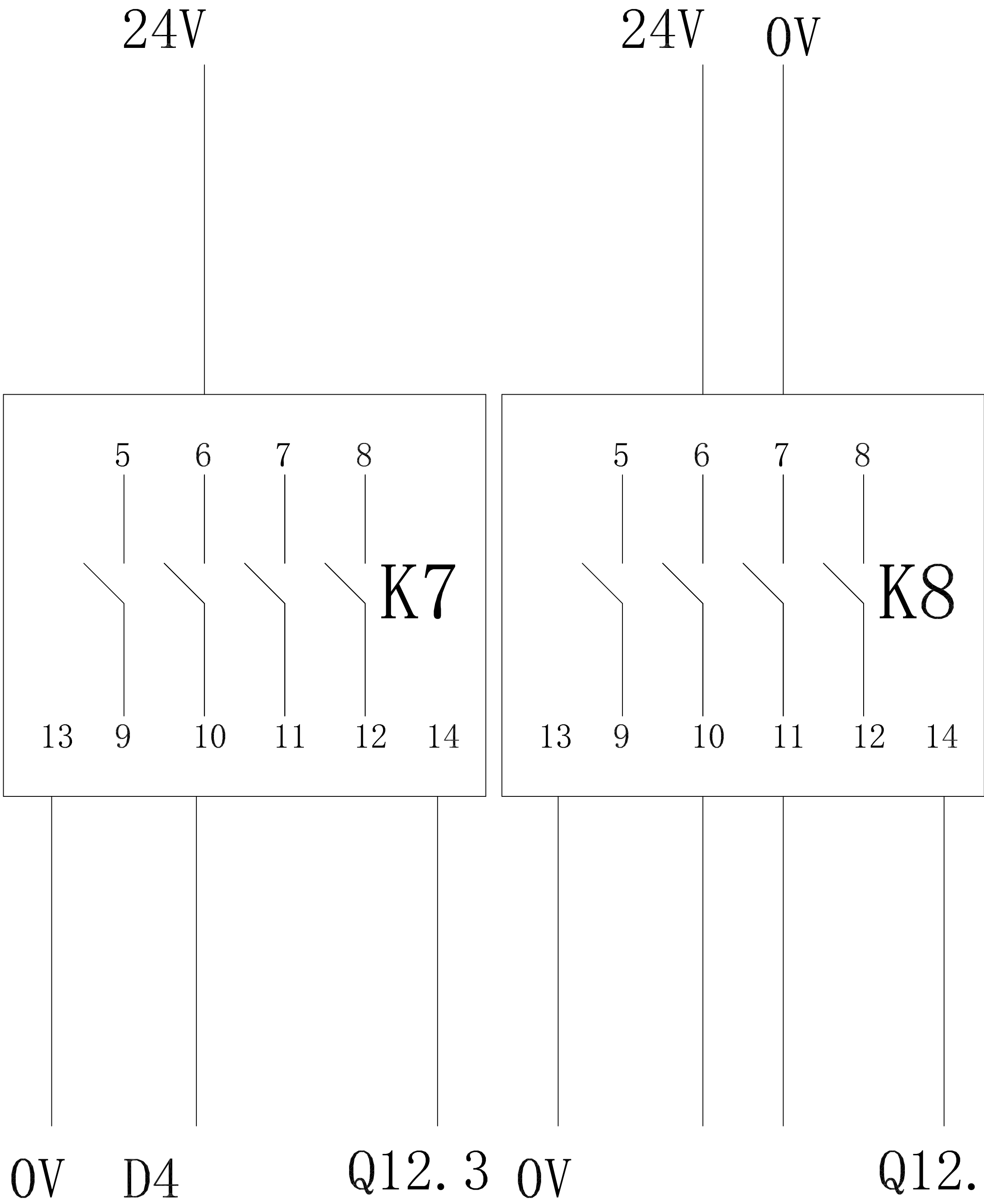
流量计电源
